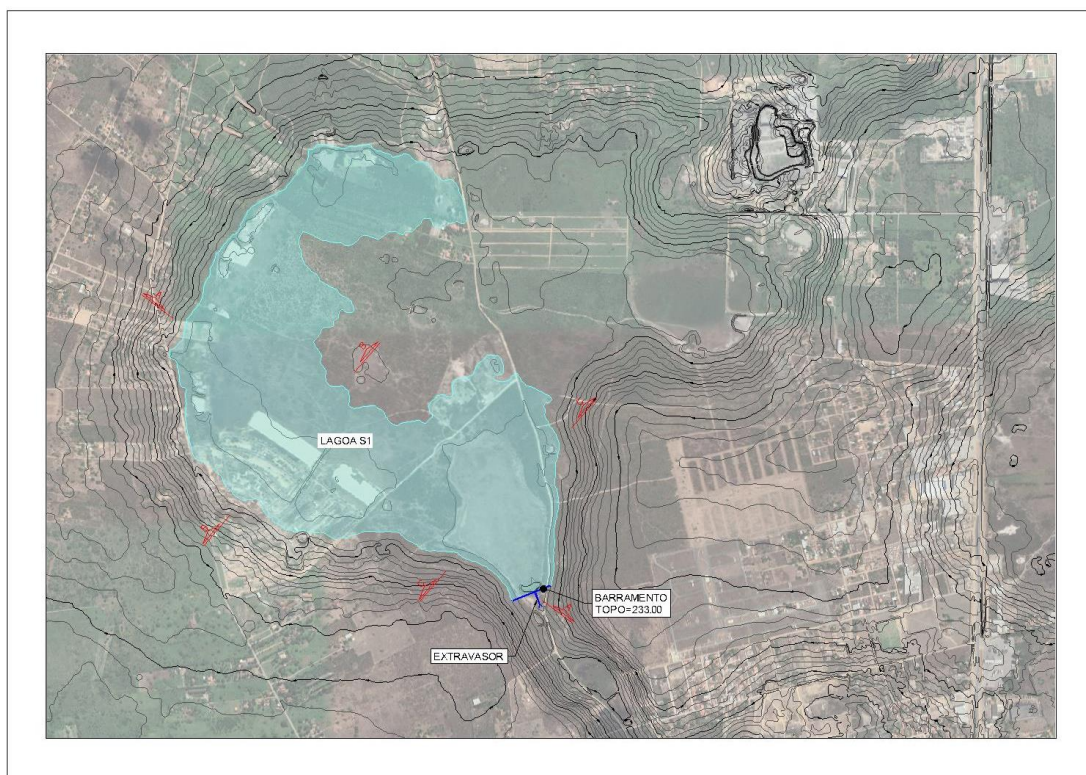
Figura 17 - Caracterização da bacia de retenção da Lagoa S1
