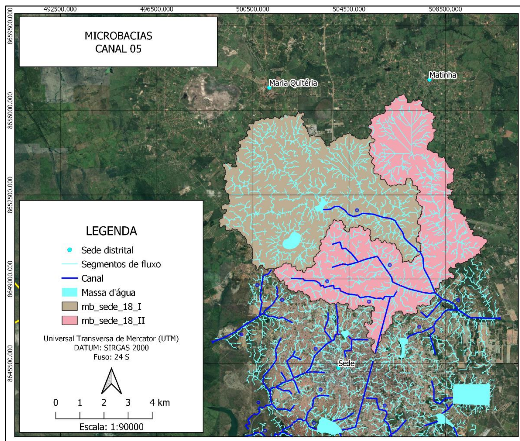
Figura 15 - Caracterização das sub-bacias definidas para os estudos hidrológicos no Canal 05
