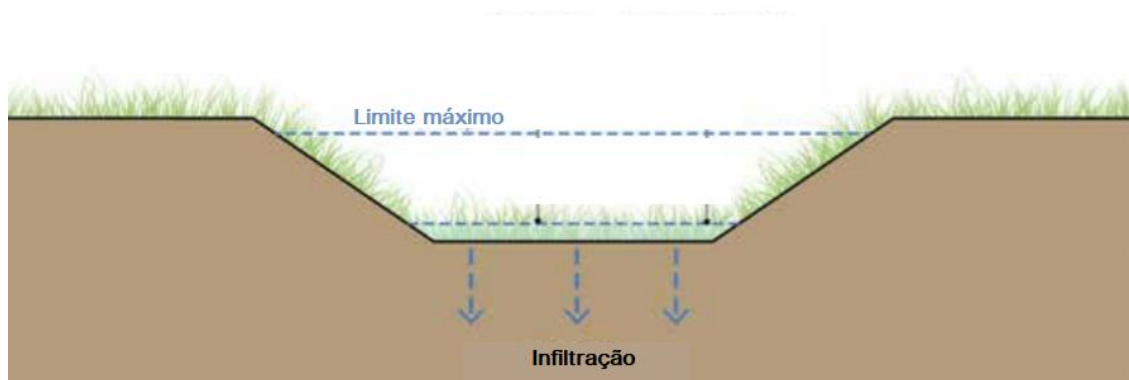
Figura 78 - Esquema típico de uma vala
