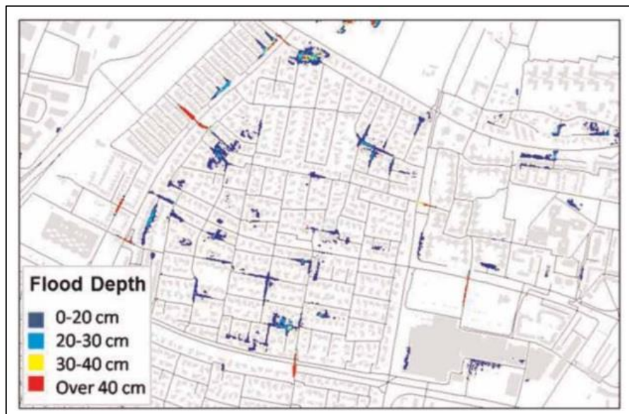
Figura 27 – Mapeamento de profundidade de inundações a partir de modelo hidrológico.
