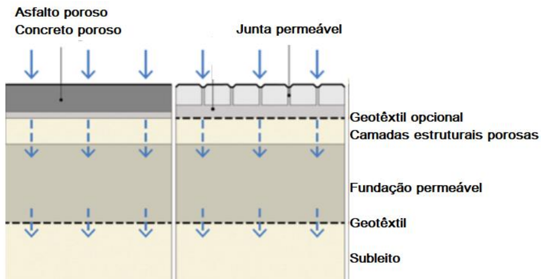
Figura 67 - Esquema de pavimento permeável com infiltração total
