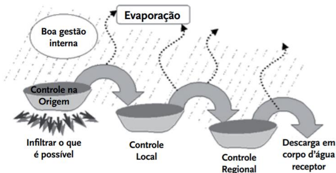
Figura 63 - A hierarquia das medidas não convencionais de controle pluvial
