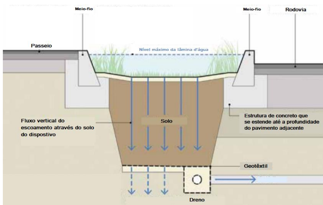
Figura 77 -Sistema de biorretenção projetado para evitar a infiltração da água na sub-base do pavimento
