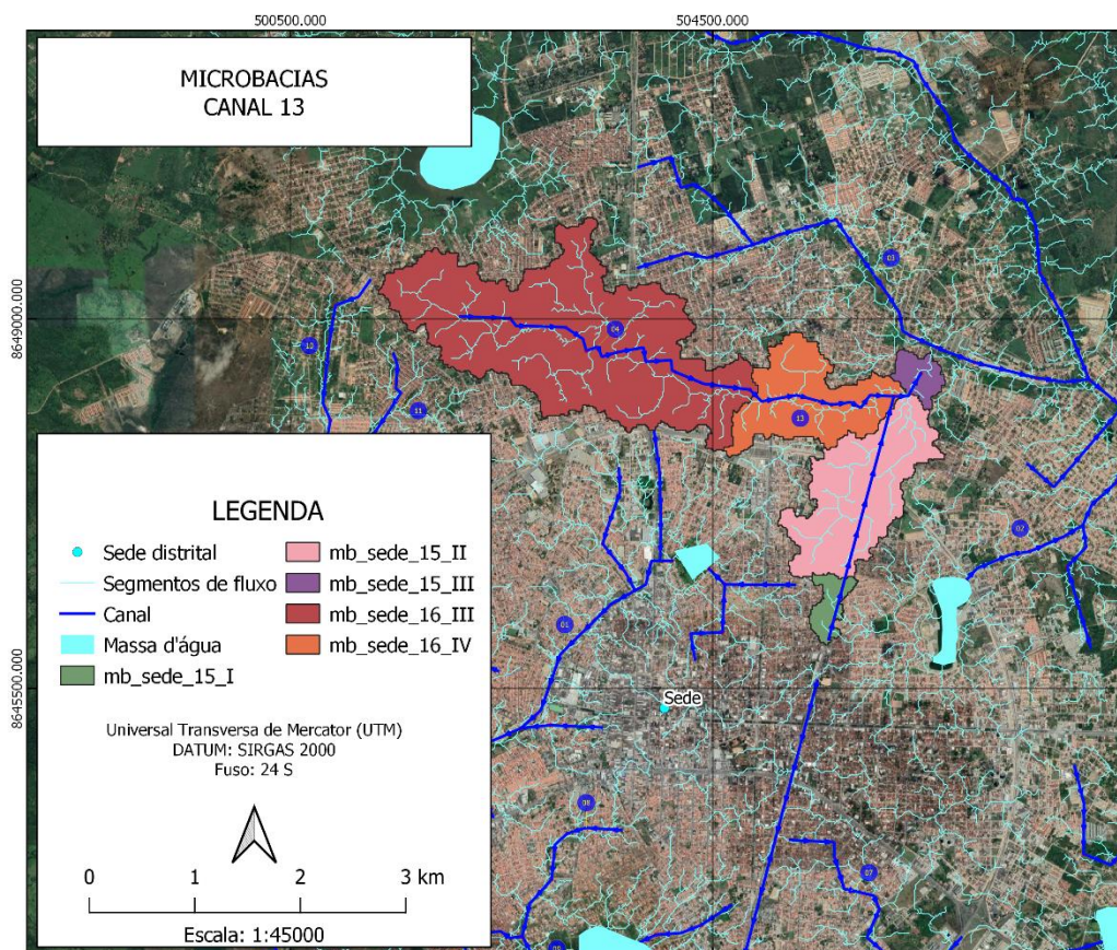
Figura 11 - Caracterização das sub-bacias definidas para os estudos hidrológicos
