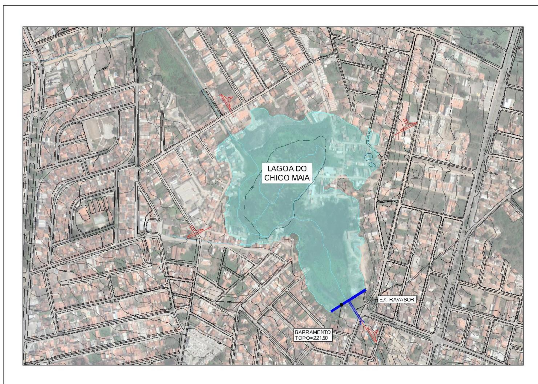
Figura 7 - Caracterização da bacia de detenção da Lagoa do Chico Maia
