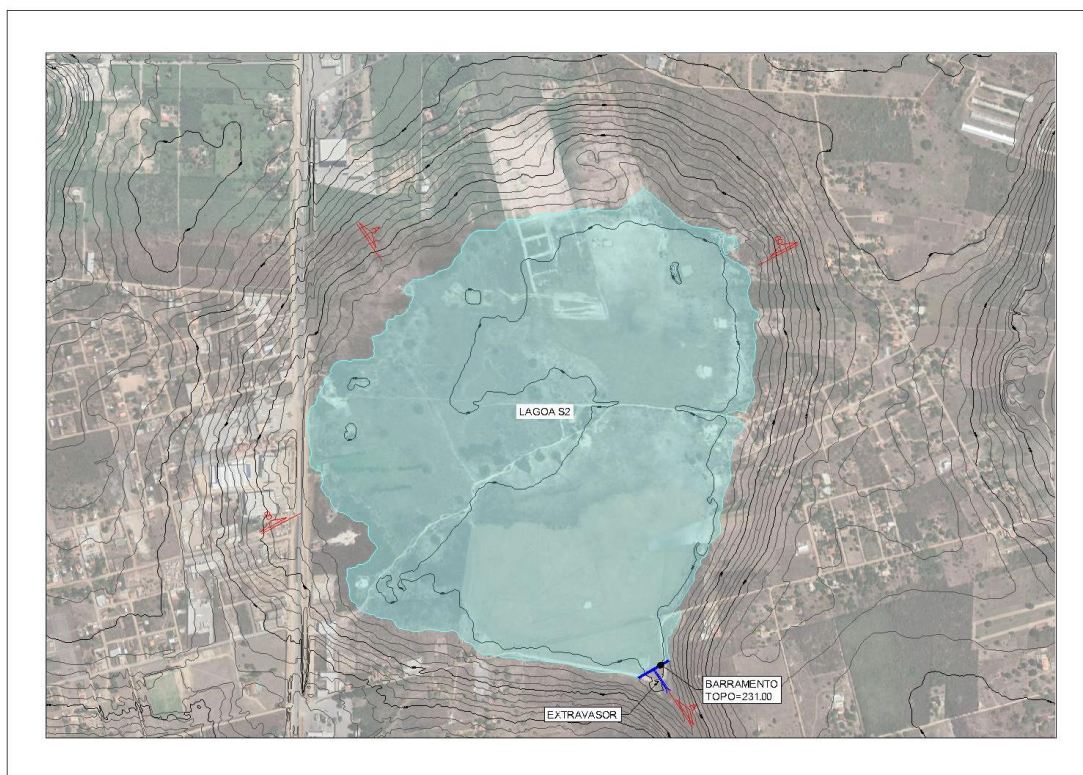
Figura 23 - Caracterização da bacia de retenção da Lagoa S2
