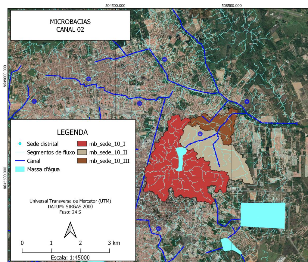
Figura 3- Caracterização das sub-bacias definidas para os estudos hidrológicos e localização da Lagoa Grande
