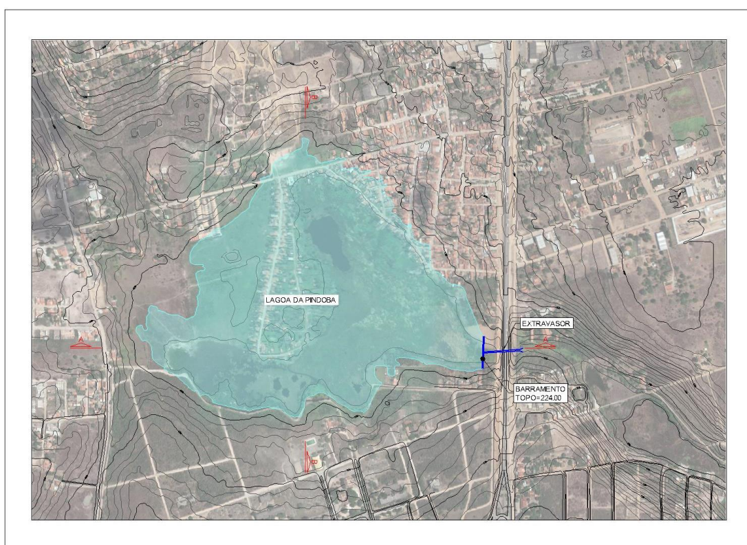
Figura 21 - Caracterização da bacia de detenção da Lagoa da Pindoba
