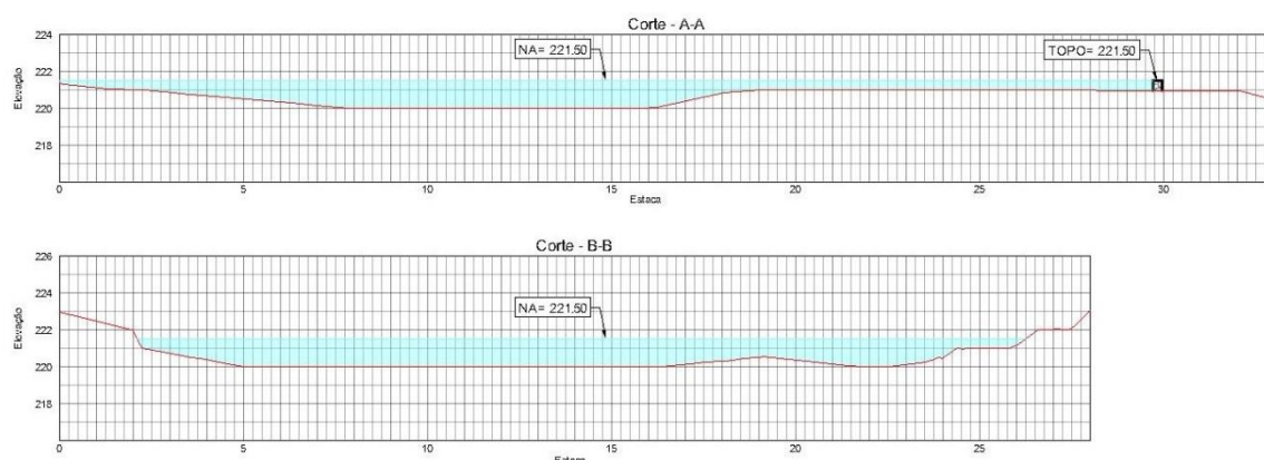
Figura 8 - Seções de terraplenagem da Lagoa do Chico Maia
