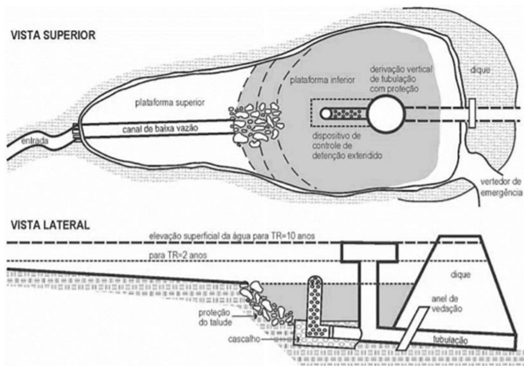
Figura 75 - Esquema do reservatório de detenção aberto
