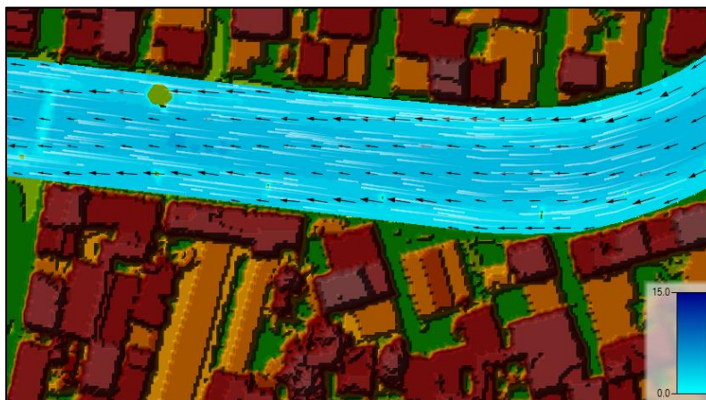
Figura 46 - Exemplo de Simulação Teste em Software SWMM
