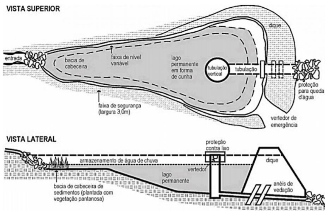
Figura 74 - Esquema do reservatório de retenção aberto
