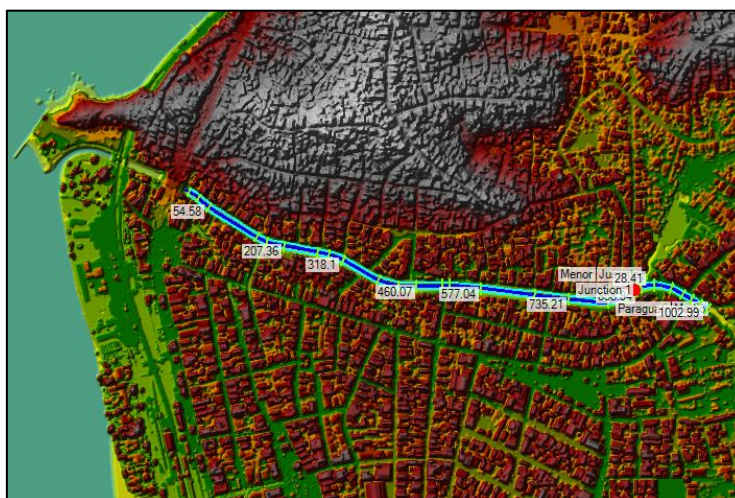
Figura 45 - Exemplo de Modelo Digital de Superfície
