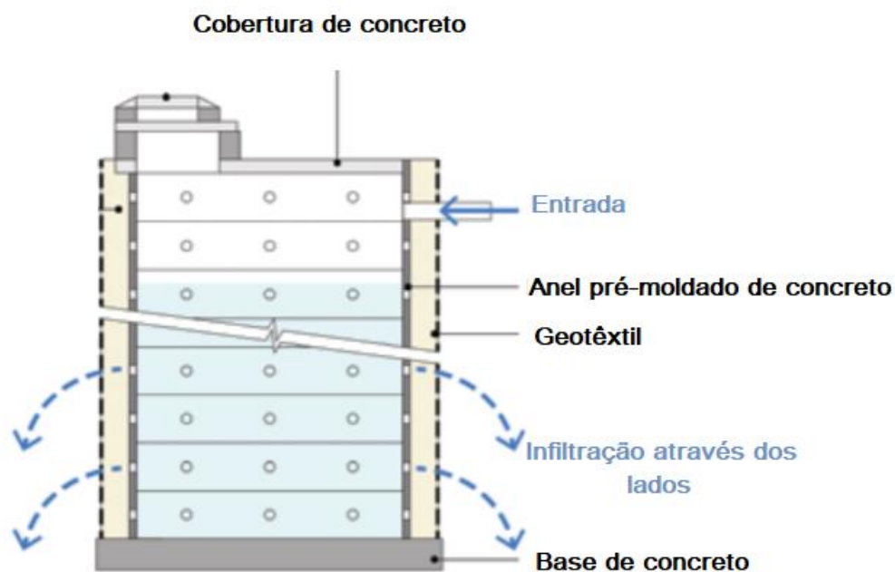
Figura 66 - Esquema de um poço de infiltração
