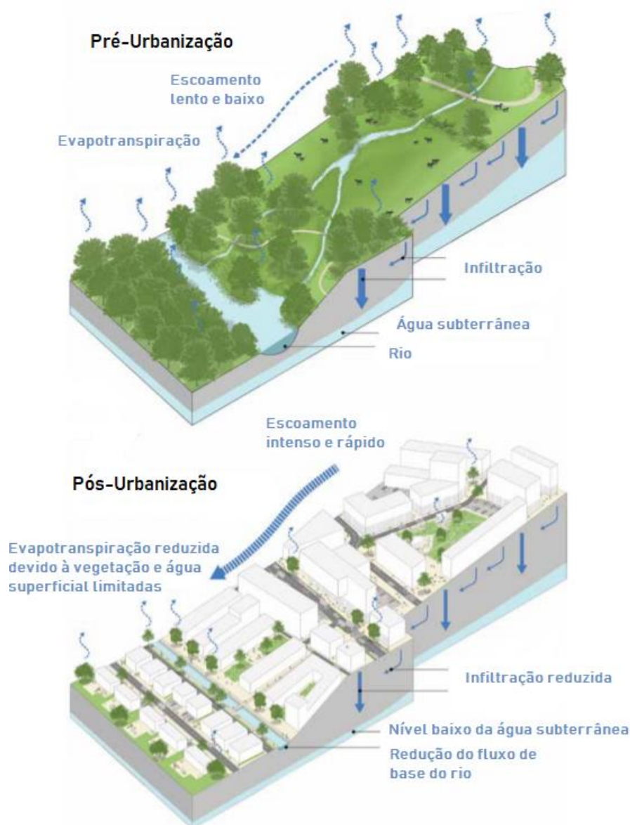
Figura 61 - Comportamento das bacias de pré-urbanização e pós-urbanização
