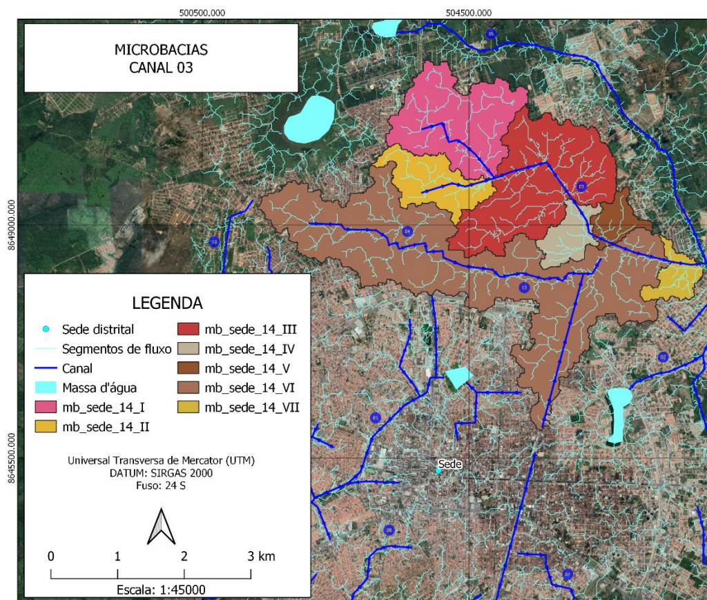
Figura 6 - Caracterização das sub-bacias definidas para os estudos hidrológicos e localização da Lagoa do Chico Maia
