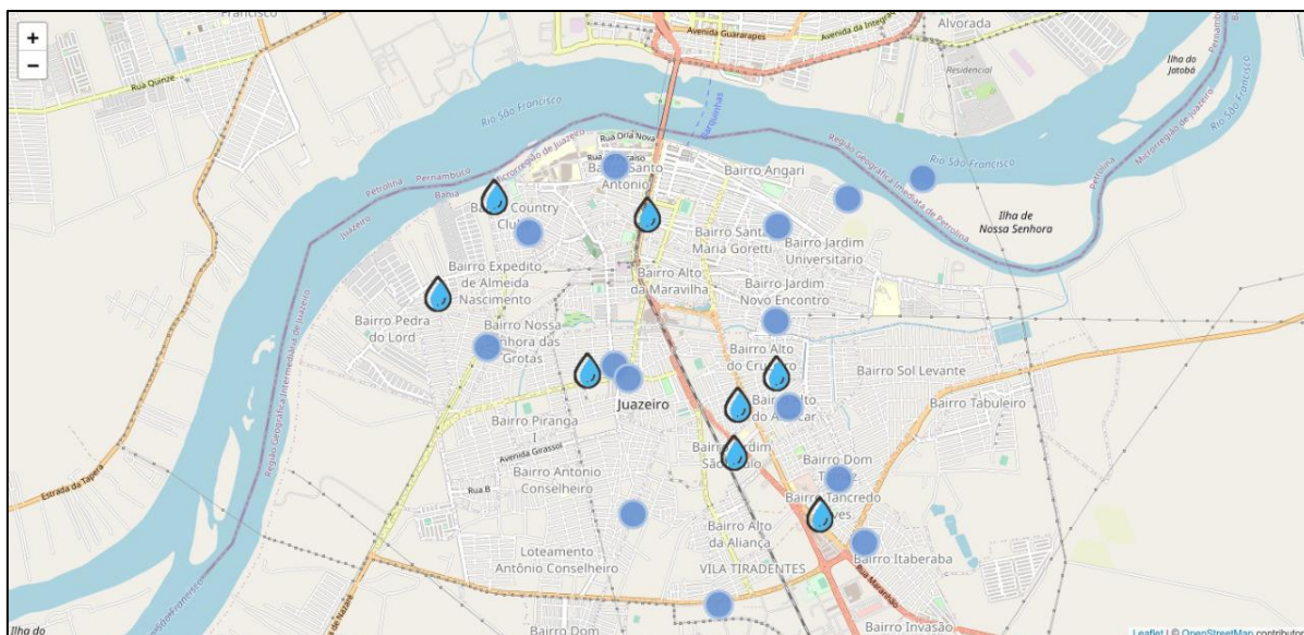
Figura 50 - Exemplo de Locais de Instalações Solicitadas (círculo azul) e Configuração dos pontos para Recebimento de Sinais (gota d'água)
