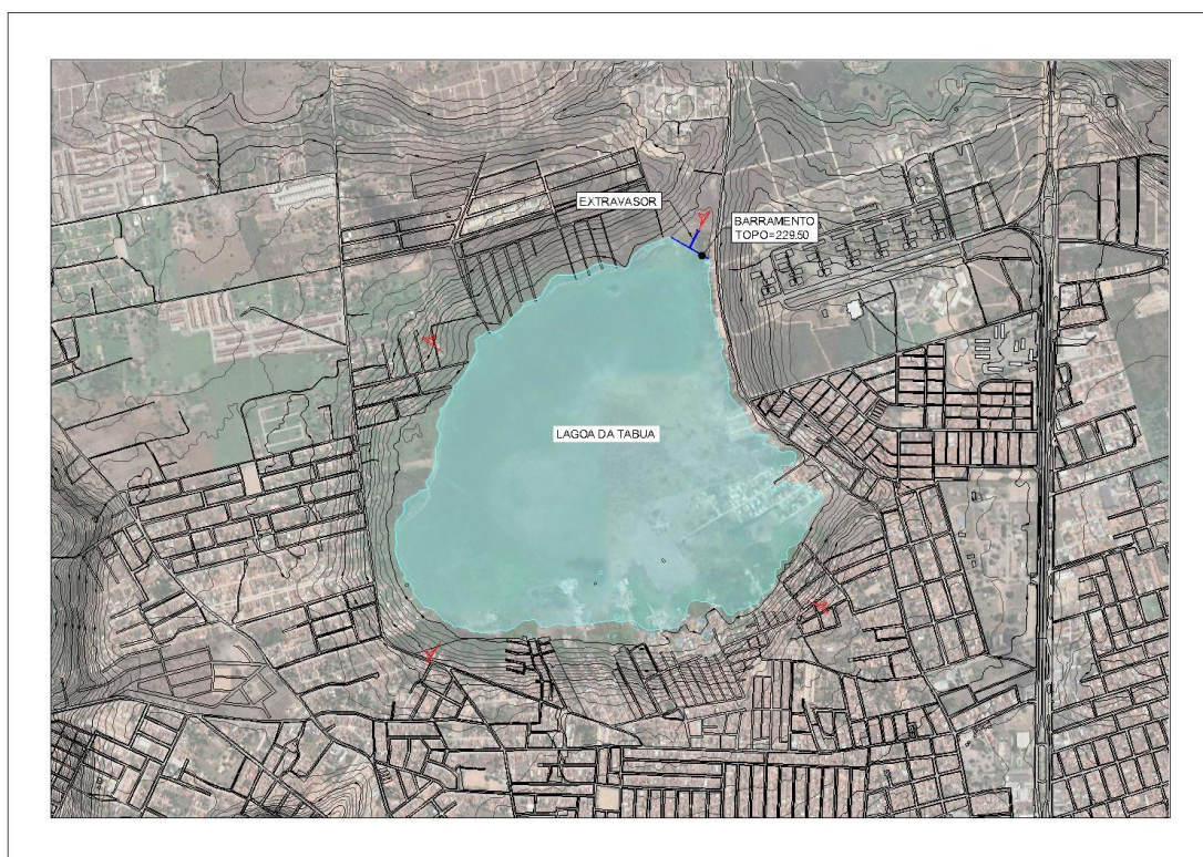
Figura 19 - Caracterização da bacia de detenção da Lagoa da Tabua
