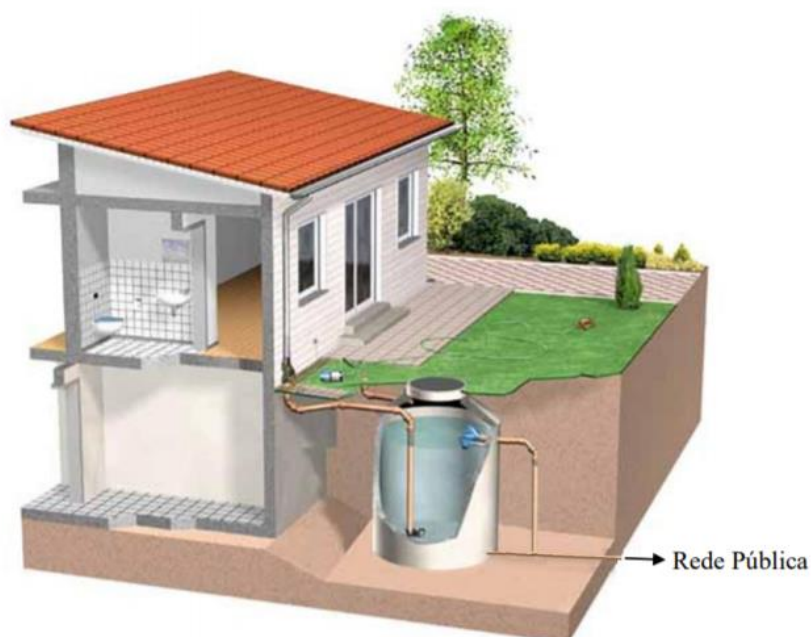
Figura 76 - Microrreservatório implantado em uma residência
