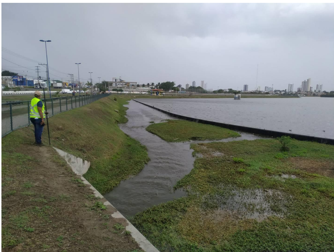
Figura 2 - Visão geral do reservatório da Lagoa Grande
