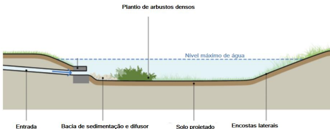
Figura 70 - Vista lateral de uma bacia de infiltração
