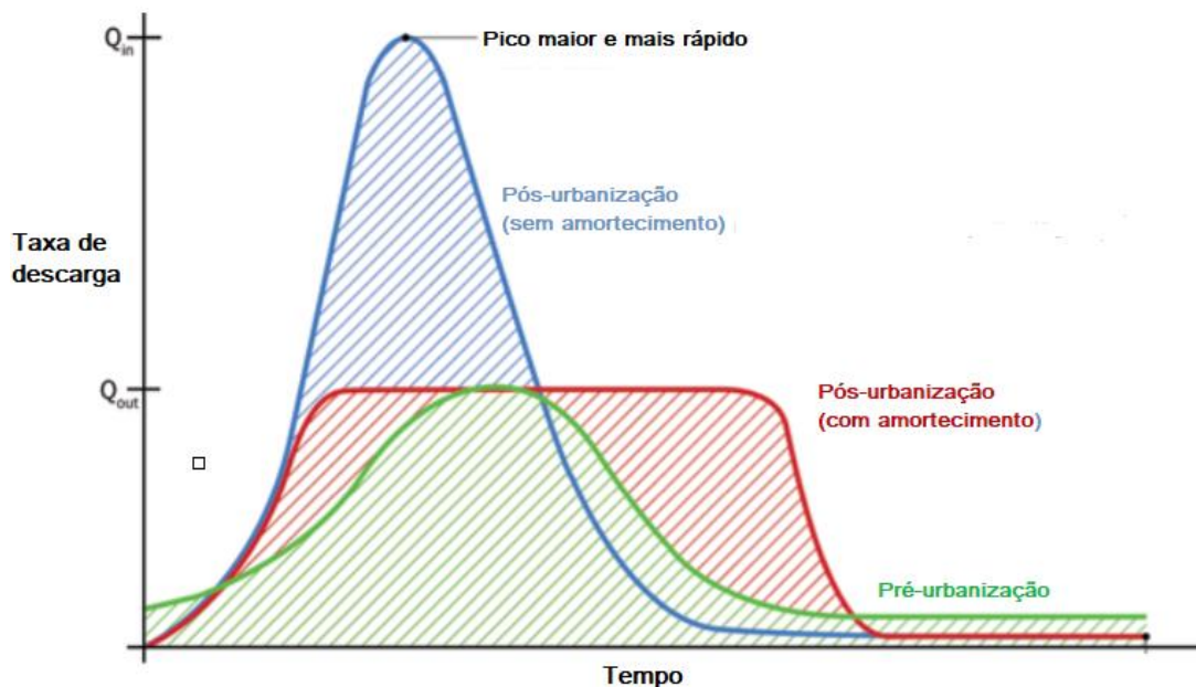
Figura 62 - Efeito da urbanização e amortecimento sobre os hidrogramas
